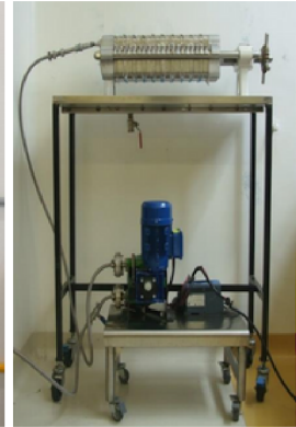
FILTRO PRENSA
